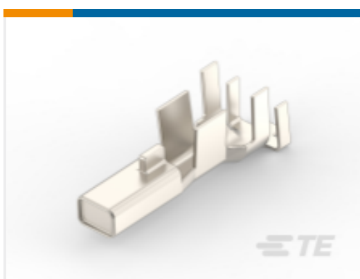
TE 产品编号 1971779-2 PTL RECEPTACLE CONTACT, 12 AWG
