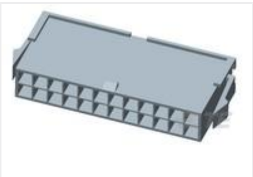
TE 产品编号1969599-2 2P PM PLUG VAL-U-LOK V2
