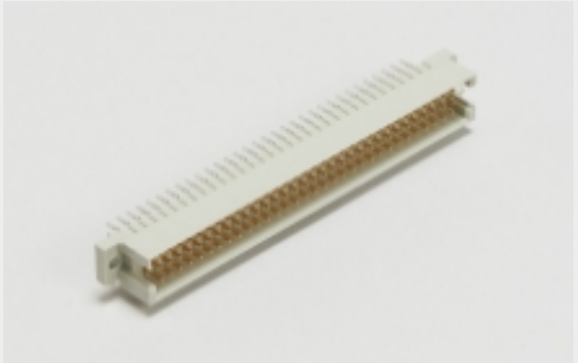
Eurocard 连接器(1)
