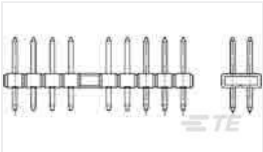
TE 产品编号 1-5176264-4 AMPMODU 2MM V 30P AU:0.2 BLACK
