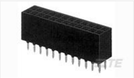
TE 产品编号1-534236-6 32 MODII VRT DR CE 100/120
