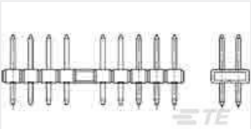
TE 产品编号 1-966926-0 2X10P MODU 2MM PIN HDR,SMD, BLSTR
