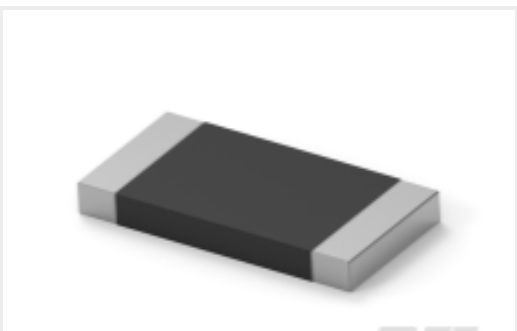
TE 产品编号4-2176422-2 TLRP 2512 3.0W R100 1% 25PPM 4K RL
