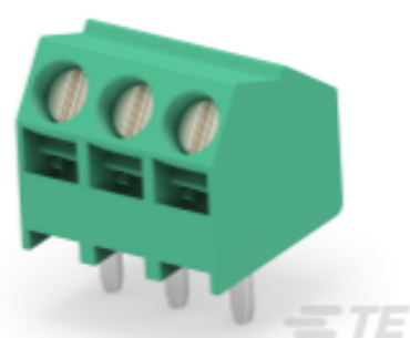
TE 产品编号 1546556-3 3P,STACKABLE,55 DEG,3.5MM
