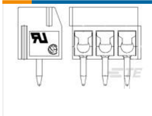
TE 产品编号1-1776275-0 10P TB ,90deg,VT,3.5mm,Blue,w /interlock
