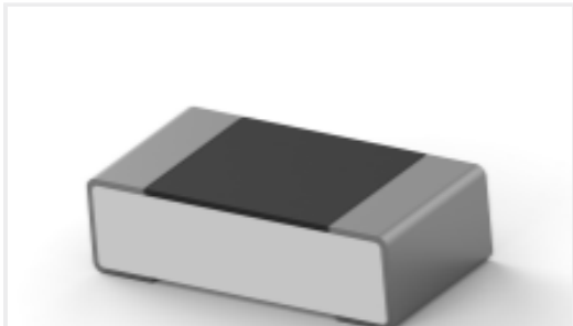
TE 产品编号1-2176369-0 RQ 0603 49R9 0.1% 10PPM 5K RL
