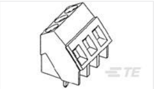
TE 产品编号796690-2 TERMI-BLOK PCB MOUNT 2P
