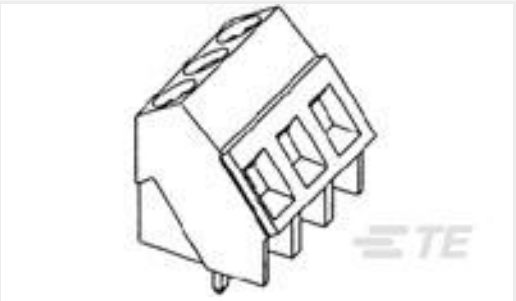
TE 产品编号796690-3 TERMI-BLOK PCB MOUNT 3P
