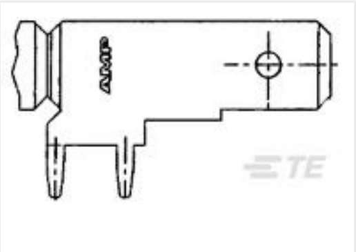
TE 产品编号63951-1 250 FASTON TAB TPBR
