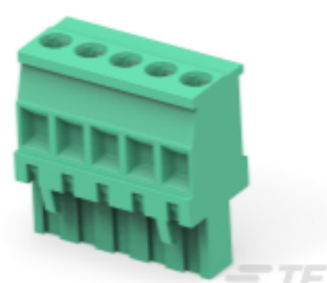
TE 产品编号 284046-5 TERMI-BLOK VERTICAL PLUG STACK
