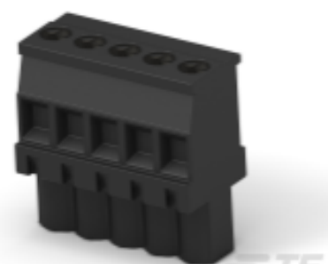
TE 产品编号 1546118-5 5 POS. 5MM VERT. PLUG LH BLCK
