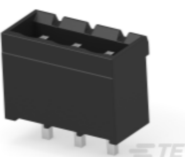
TE 产品编号 796643-3 3POS 5.0MM CE VRT HDR, TRM BLK
