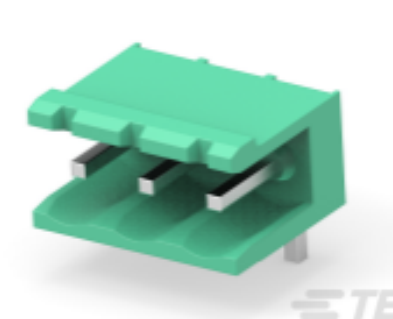
TE 产品编号 282812-3 TERMI-BLOK HEADER, ASSY 3P. 5
