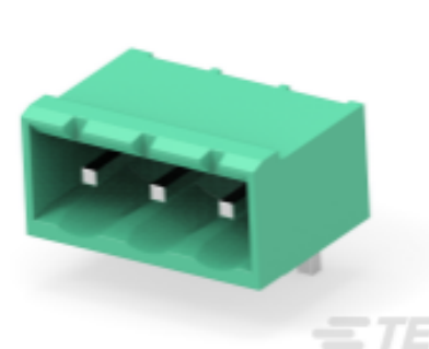
TE 产品编号 796644-3 3POS 5.0MM CE R/A HDR, TRM BLK
