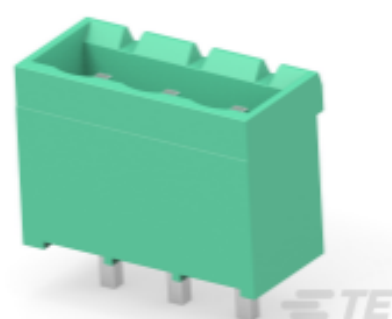
TE 产品编号 796642-3 3POS 5.0MM CE VRT HDR, TRM BLK
