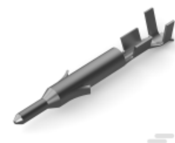
TE 产品编号 770901-1 MINI UMNL PIN 26-22 AWG SN
