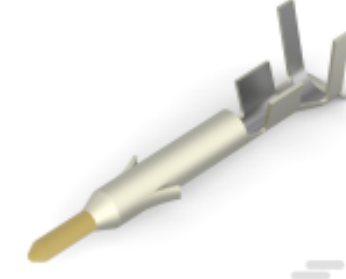
TE 产品编号 1-770903-0 MINI UMNL PIN 22-18 AWG AU
