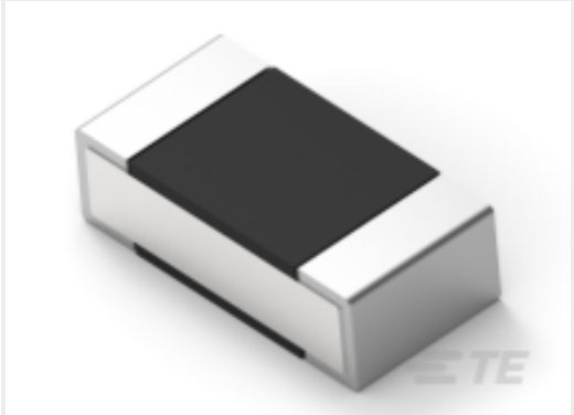
TE 产品编号4-2176307-9 RP 1E 0.1W 39K2 0.1% 25PPM 5K RL
