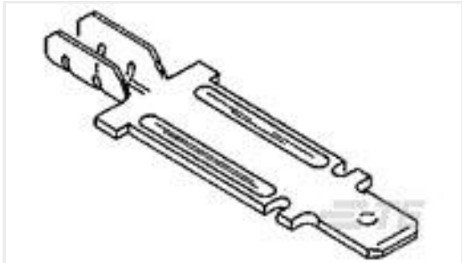
TE 产品编号63522-1 250 FASTON TAB 20-15 AWG NPST
