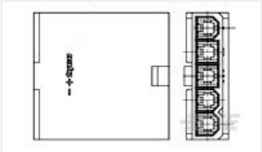
TE 产品编号1586024-5 5P S/R FH PLUG VAL-U-LOK V2
