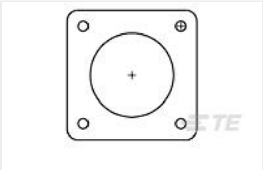
TE 产品编号81665-2 FLANGE GASKET CPC
