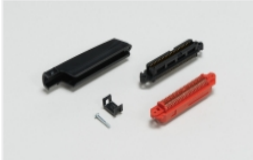
IDC D-Sub 连接器(69)
