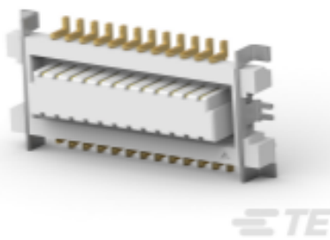
TE 产品编号1775013-2 0.8 BTB FS RCPT G/F 24P
