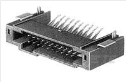
TE 产品编号5-104894-2 20 50/50 GRID RA HDR LF
