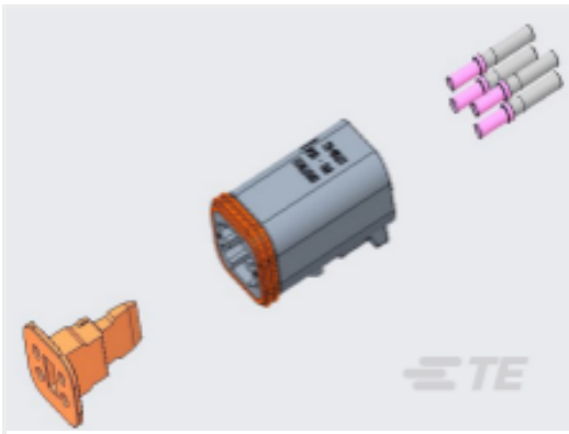
TE 产品编号DT06-4S-COMplete DT06-4S CON AND WEG
