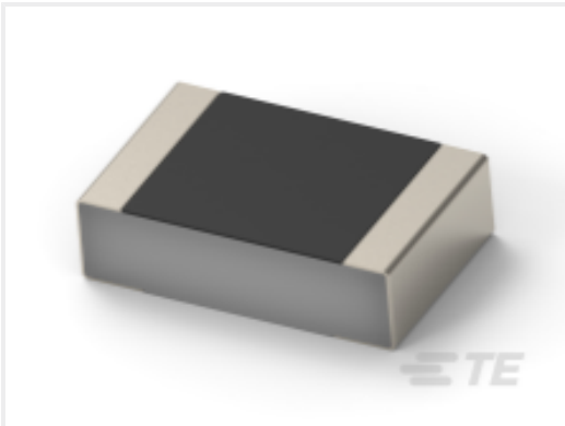
TE 产品编号9-2176452-0 CPF 0201 4K53 0.1% 25ppm 1K RL
