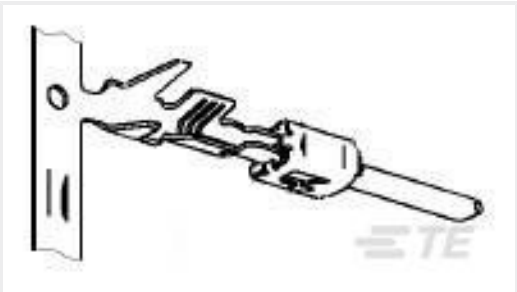
TE 产品编号2-2141598-2 TAB 2.8x0.8 CONTACT CF SRC Ag
