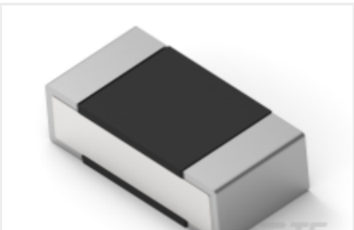
TE 产品编号9-2176312-0 RP 1E 0.1W 105K 0.1% 25PPM 1K RL
