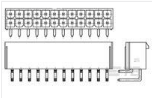
TE 产品编号2-1586041-4 24P VAL-U-LOK R/A HDR V2
