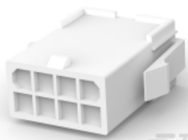
TE 产品编号 794941-1 08P MINI UMNL CAP HSG
