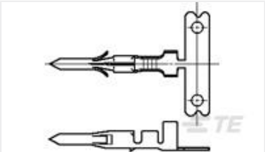
TE 产品编号350629-8 .062 COMM P&S PIN PRE TIN/PHBZ
