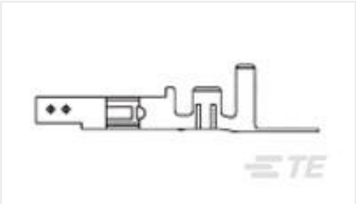
TE 产品编号794956-3 VAL-U-LOK SKT PHBZ SN 22-18AWG
