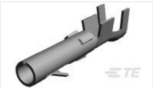
TE 产品编号61117-1 CMNL SOK 20-14 TPBR
