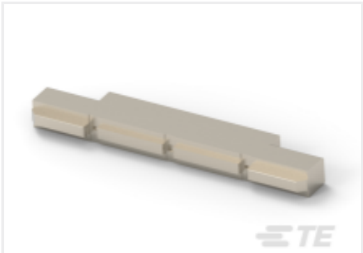
TE 产品编号767514-6 INSERTER, 228 POS. R/A PLUG
