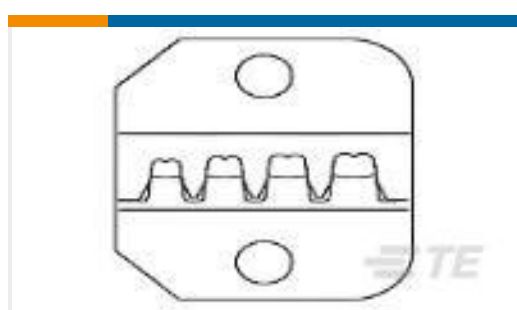
TE 产品编号58425-3 DIE, COAX 151/324X042 SQ IS9657
