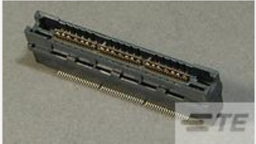
TE 产品编号 1-767153-0 114 POS. .355 VERTICAL RECEPTA
