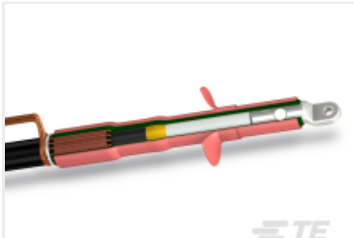
TE 产品编号 C82154-013 POLT-12D/1XO
