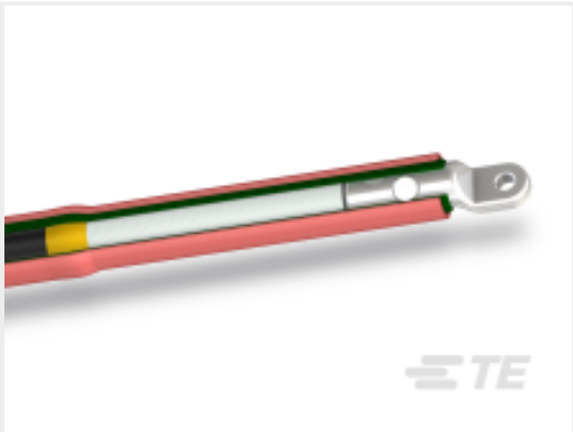
TE 产品编号CJ0364-070 POLT-24D/1XI-ML-4-13
