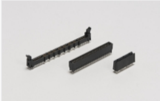
卡边缘电源连接器(1)
