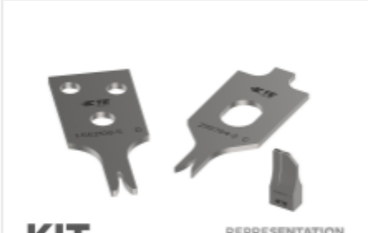
TE 产品编号7-2836636-7 OC-075F-CRIMPTOOLINGKIT
