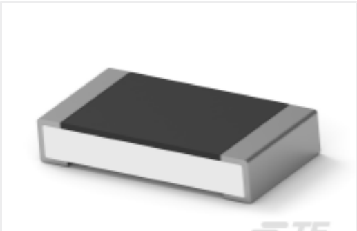
TE 产品编号4-2176384-4 RQ 1206 301R 0.1% 10PPM 1K RL
