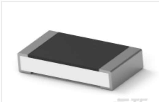
TE 产品编号4-2176386-2 RQ 1206 33K2 0.1% 10PPM 1K RL
