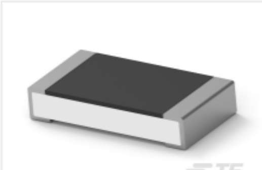
TE 产品编号2-2176387-2 RQ 1206 221K 0.1% 10PPM 1K RL
