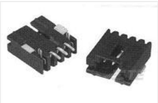
TE 产品编号5-147278-1 02 MTE HDR SRRA SFMNT .100CL
