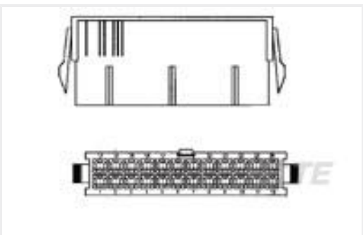
TE 产品编号2-1586018-4 24P PM PLUG VAL-U-LOK V0
