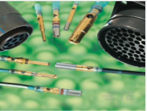
TE 产品编号946441-000 D-602-1117
