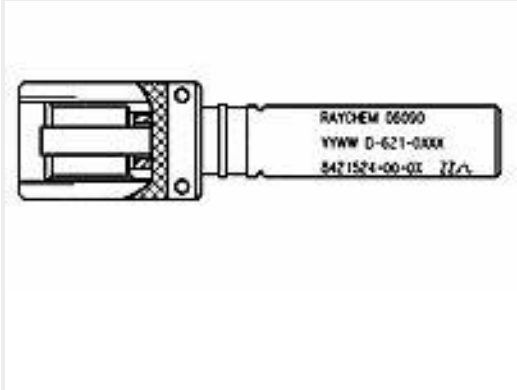
TE 产品编号435589-000 D-621-0413
