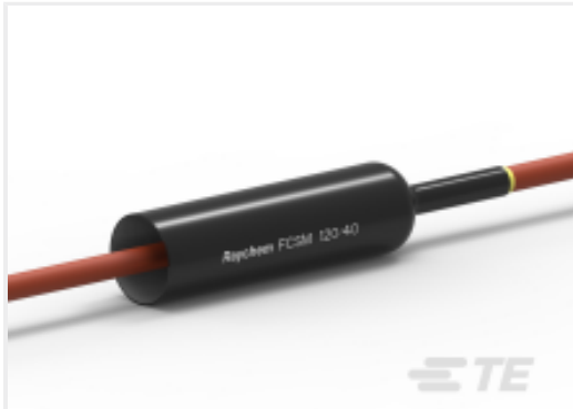
TE 产品编号 926396-000 FCSM-120/40-1500/S(S5)
