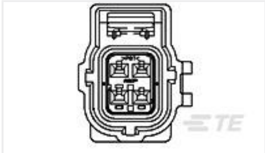
TE 产品编号184394-1 2X2 PLG ASY W/RET W/O CPA C3-A
