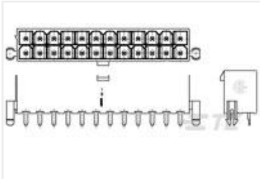
TE 产品编号1586039-2 2P VAL-U-LOK VRT HDR W/P V2
