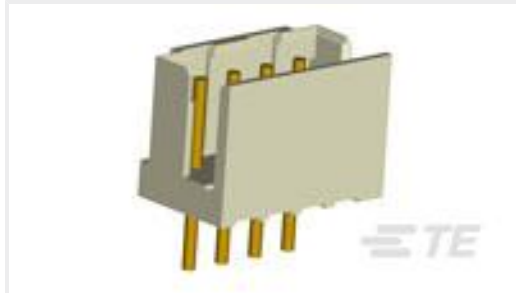
TE 产品编号 7-292165-5 CT P/HDR BOX V 15P T/P BLACK
