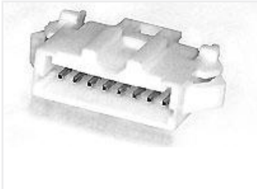
TE 产品编号1-292215-0 MINI CT SGL RELAY 10P NAT
