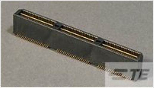
TE 产品编号 7-1658465-3 MSB0.80PL11ASY84DP,GP,30,VCTR
