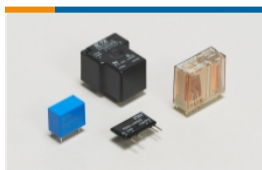
功率继电器(106)
