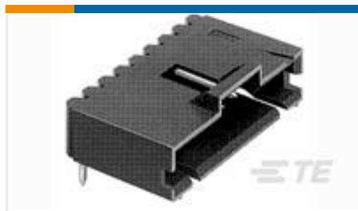
TE 产品编号 7-104935-4 25 MTE HDR SRRA LTCH.100CL LF
