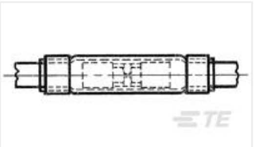
TE 产品编号324370 SPlice,PO INS BUTT 26-24 KIT
