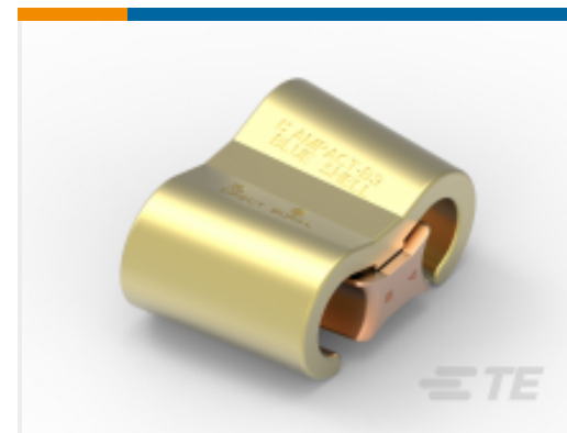
TE 产品编号 276337-3 AMPACT CU TAP 450-2/0
