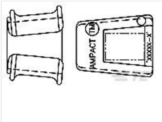
TE 产品编号602283 AMPACT AI Tap 1/0-2
