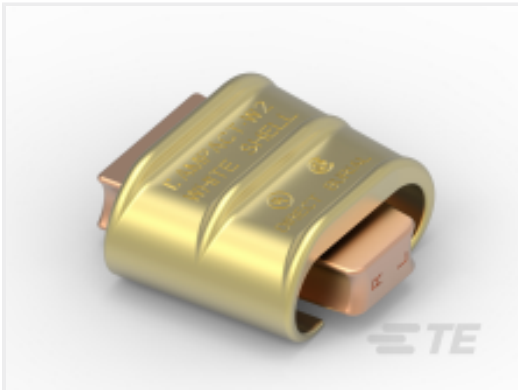
TE 产品编号 275187-3 AMPACT CU TAP 250-2/0
